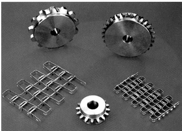
Nastri grecati e ingranaggi "Grecati" belts and sprockets
