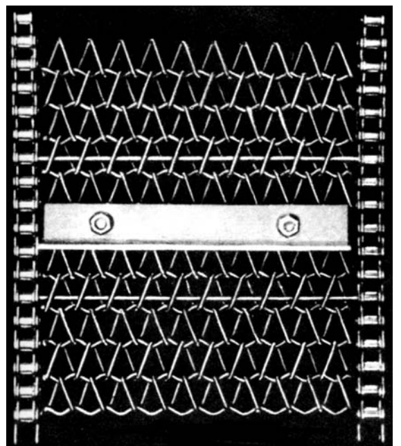
NC: con catene calibrate ai lati - vengono montati anche con arresti per il trasporto inclinato with calibrated chains at the sides - available also with entrainers for the sloping conveyance
